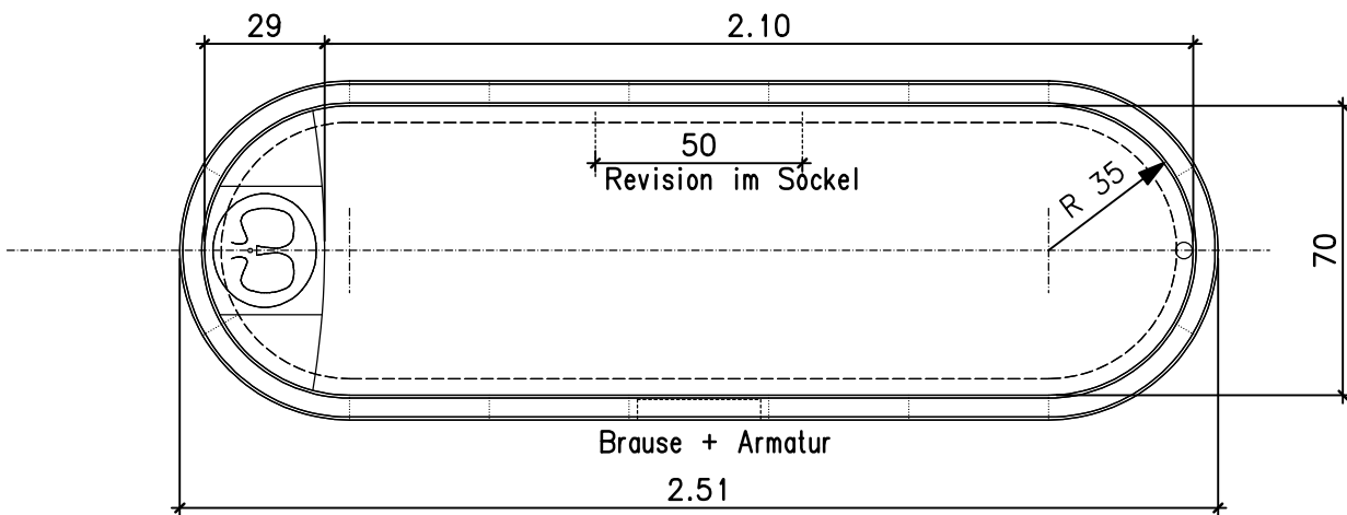
Grundriss
